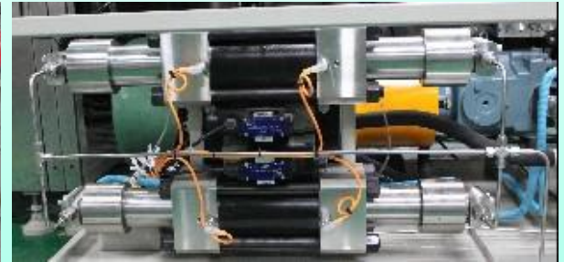
内部结构
